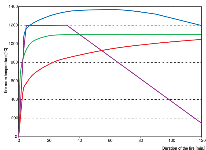
Curva de temperatura: — (ETC), — Curva de Hidrocarboneto, — RABT/ZT — Rijkswaterstaat
